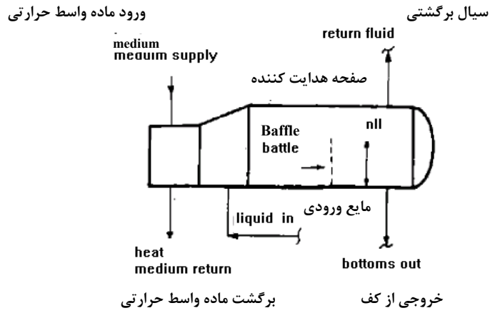
kettle type reboiler u tube type (general configuration) باز جوشاننده لوله U شکل نوع کنری (شکل عمومی)
